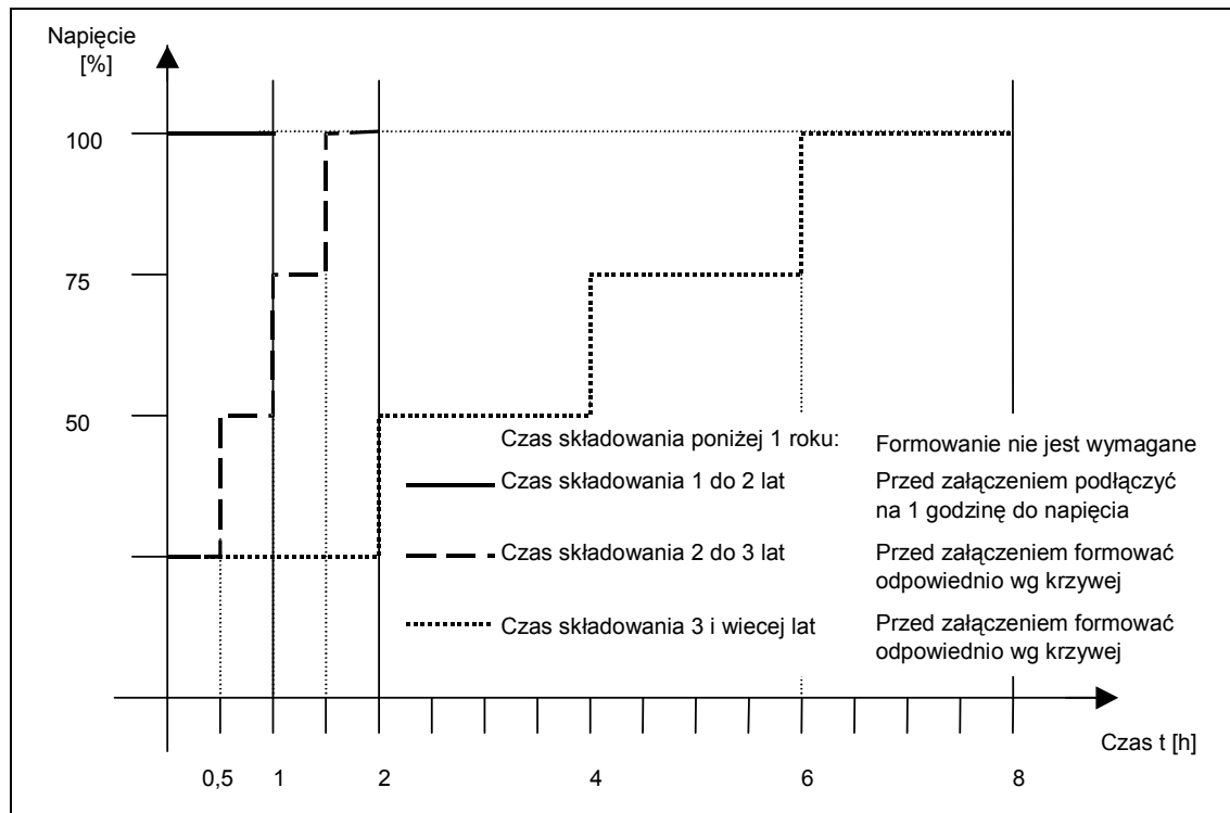
Rys. 2-1 Formowanie
