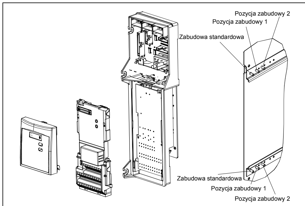
Rys. 2-7 Opcje dla kasety elektroniki
