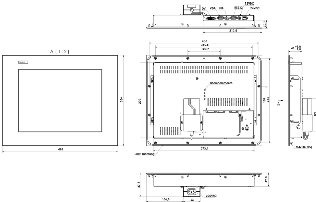
Abb. 1: Abmessung des SCD 1597-E(ET)
