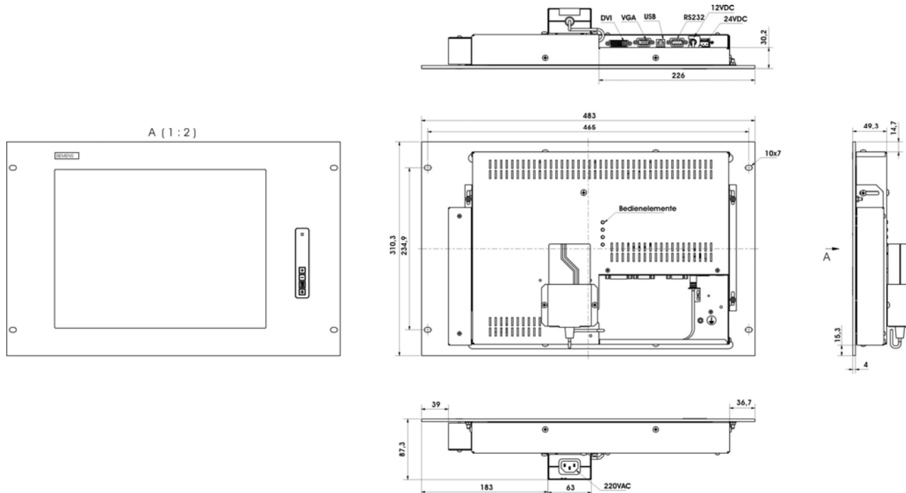
Abb. 2: Abmessung des SCD 1597-R(RT)
