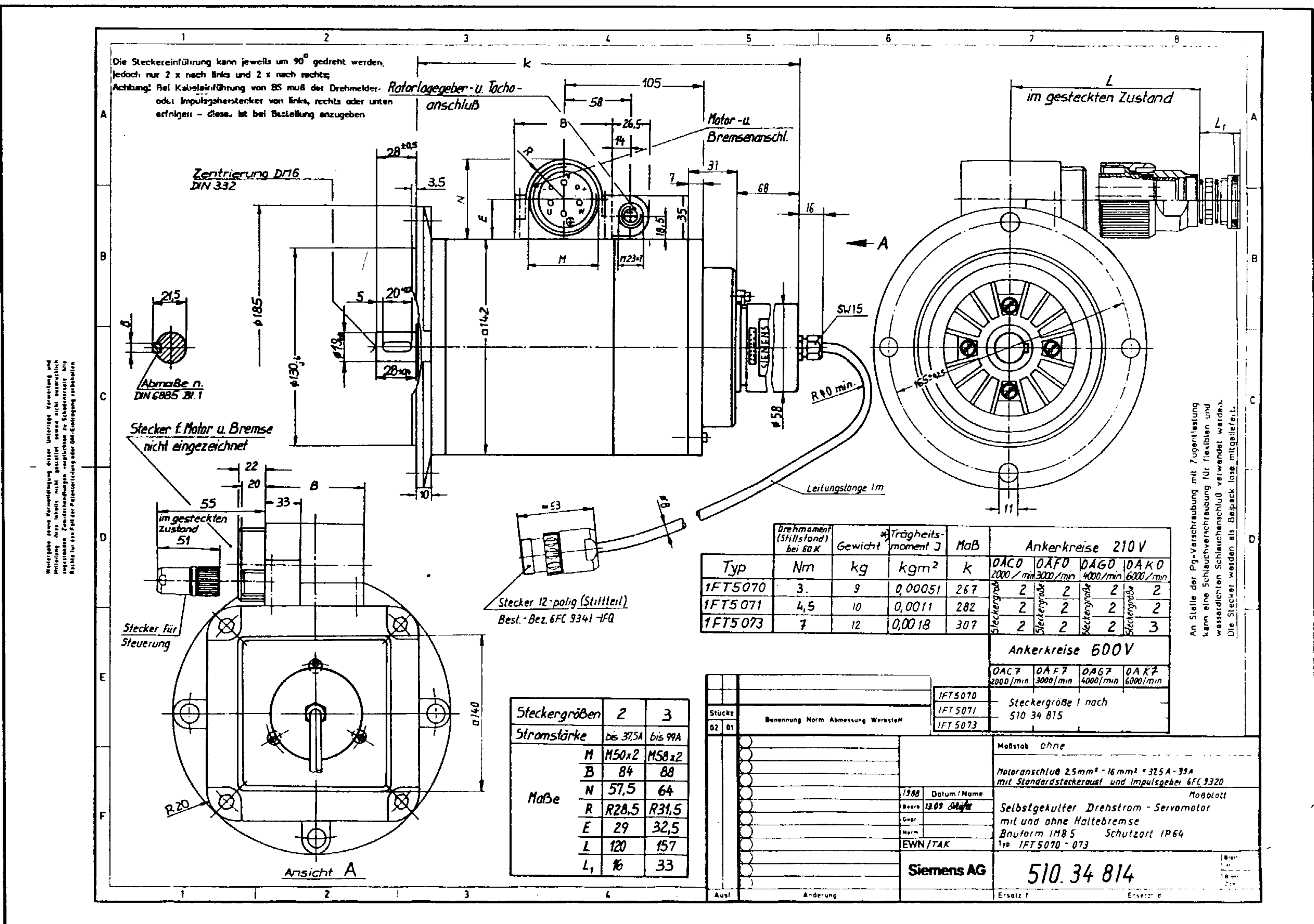
Bild 6.51 Maßblatt Drehstrom-Servomotoren 1FT5070, 1FT5071 und 1FT5073 mit Option Steckerausführung Bauform IM B5
