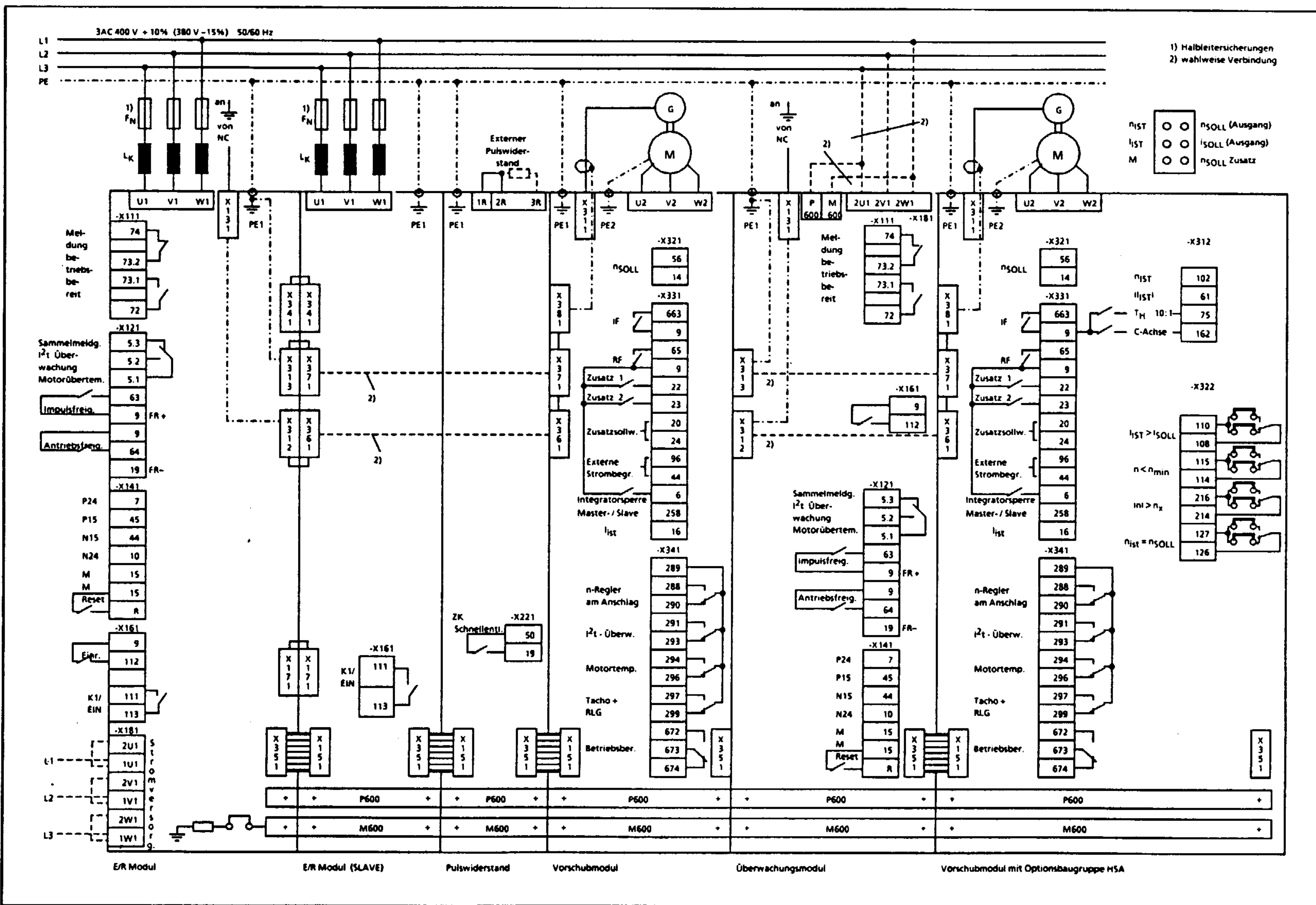
Bild 5.11 Anschlussvorschlag Pulsrichter 6SC611
