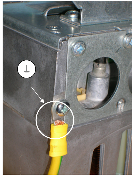
Rysunek 6-15. Podłączenie dodatkowego przewodu uziemiającego, MF4. Patrz rozdział 1.3.
