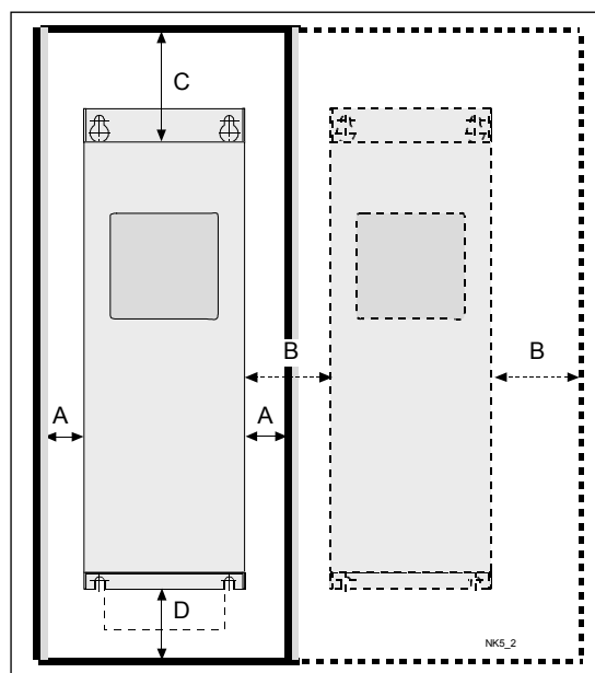
Rysunek 5-6. Przestrzeń montażowa
