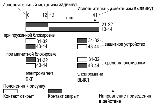
Рисунок 2: Виды блокировки
