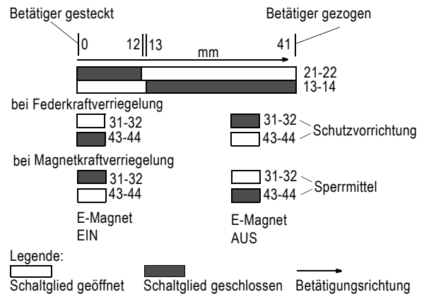
Bild 2: Verriegelungsarten
