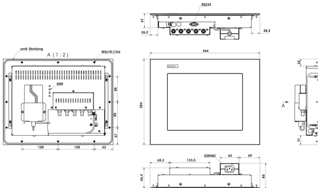
Abb. 1 Abmessung des SCD 1215-E
