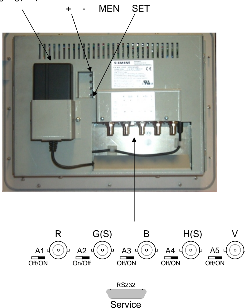
Abb. 2: Lage der Schnittstellen und Bedienelemente des SCD 1215- E
